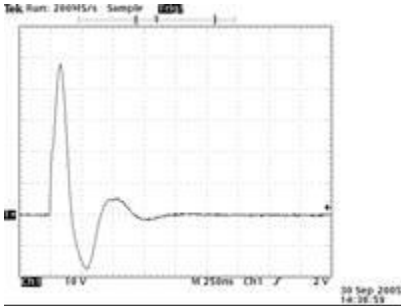
C=500pF/R=0Ω
