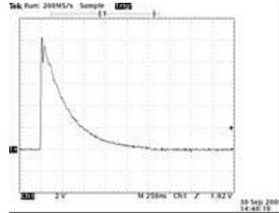
C=500pF/R=500Ω
