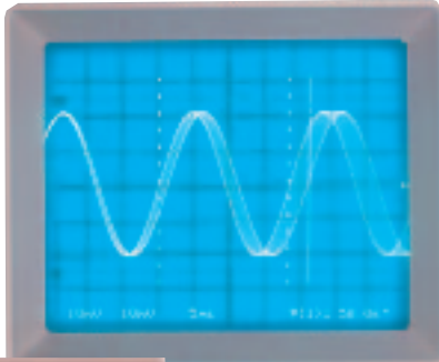
Analogdarstellung einer Frequenzmodulation
