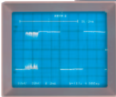
Digitaldarstellung eines vor dem Triggerpunkt liegenden transienten Störsignals
