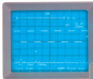
Anzeige des Signals und der zugehörigen FFT
