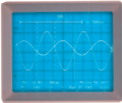
Mess cursoren und automatische Messung der Phasenlage
